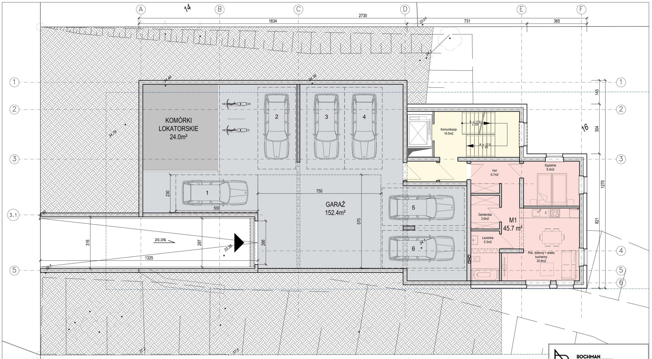
RZUT POZIOMU -1
